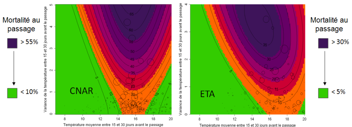
Figure 27 : Cartographie des températures à risque issue du modèle linéaire généralisé
